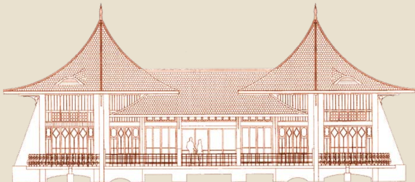
湖心亭立面示意圖
